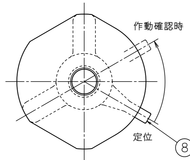
矢視 A-A 図
