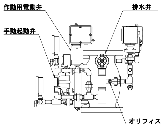
右側面図
