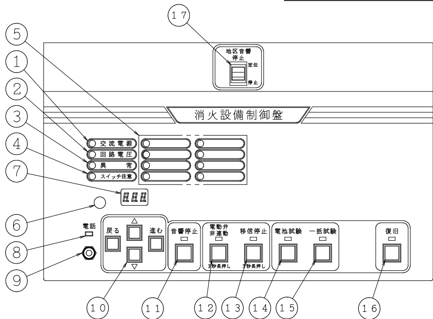
詳細図
