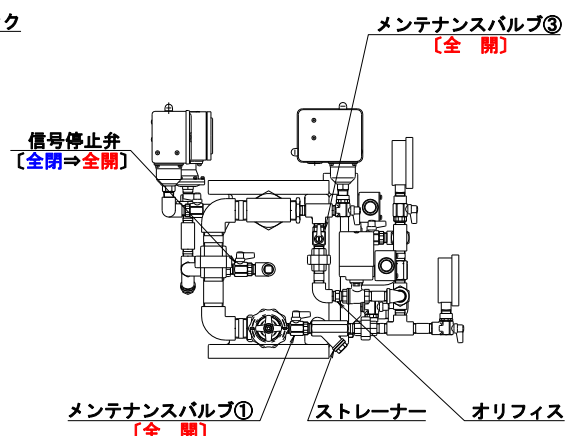
左側面図
