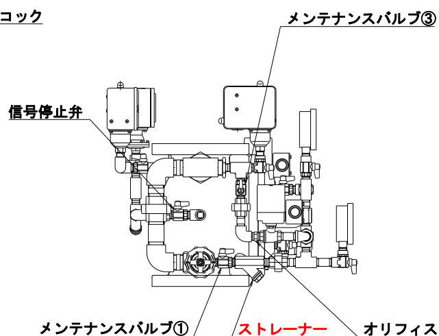
左側面図
