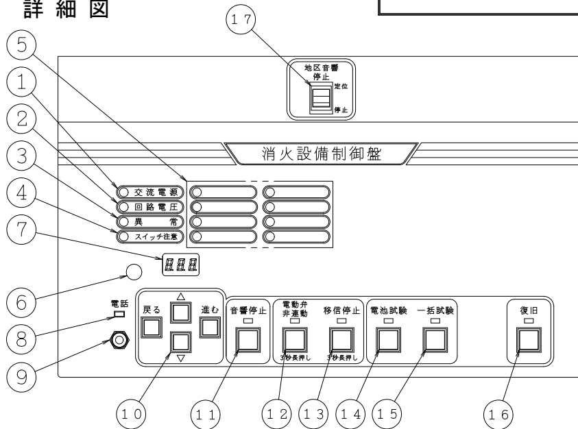
詳細図
