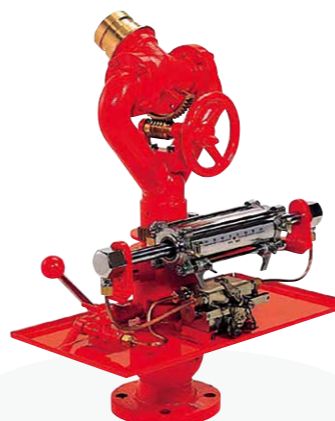
自動回転 放水銃
