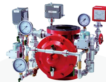
予作動式 (湿式) 流水検知装置
